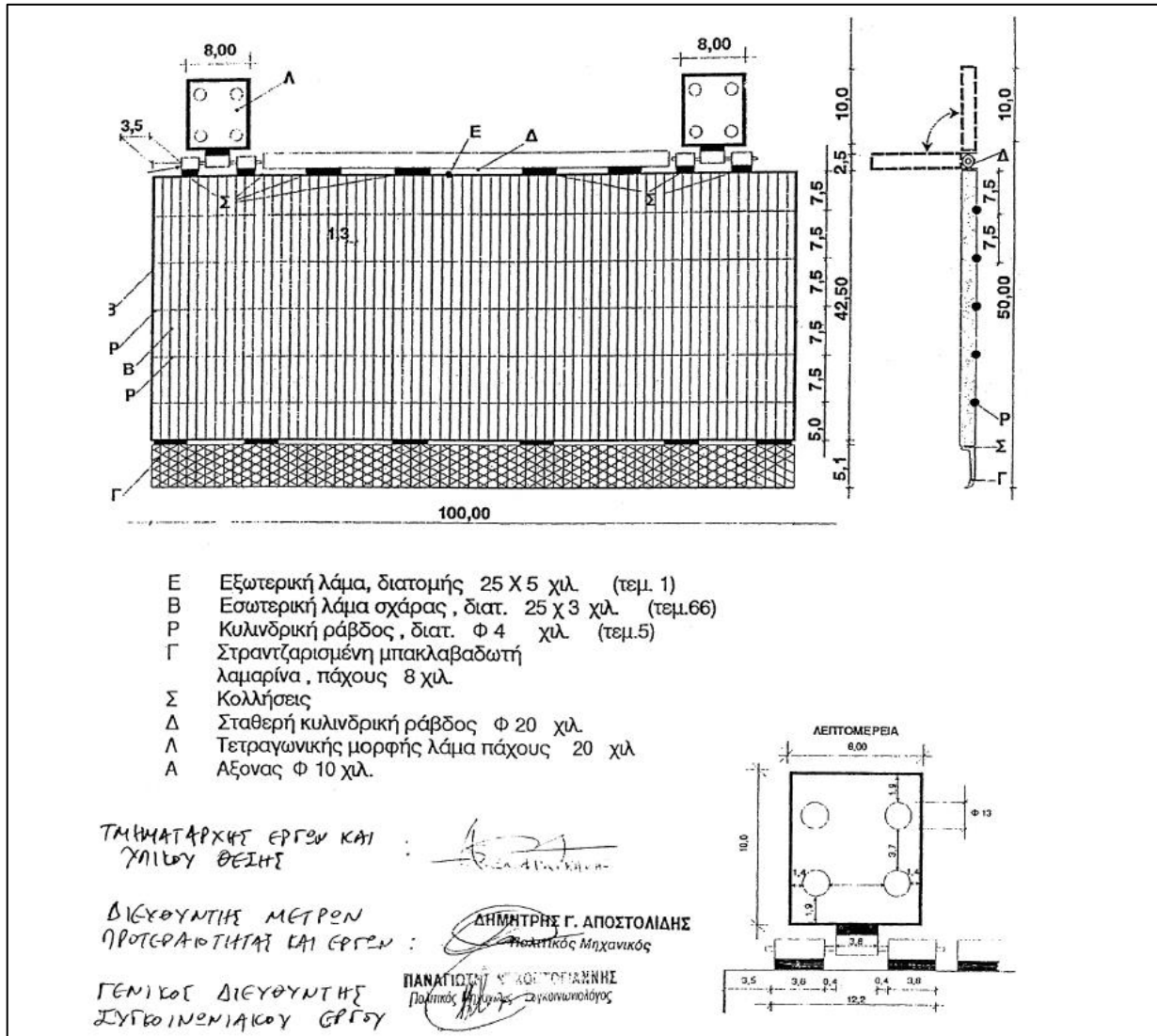
Εικόνα 1: Σχέδιο Κάτοψης Μεταλλικής Εσχάρας Σύνδεσης της Προεξοχής με το Πεζοδρόμιο
